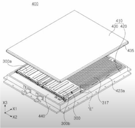
그림 24. SKOn CTP 관련 특허: 팩 구조
