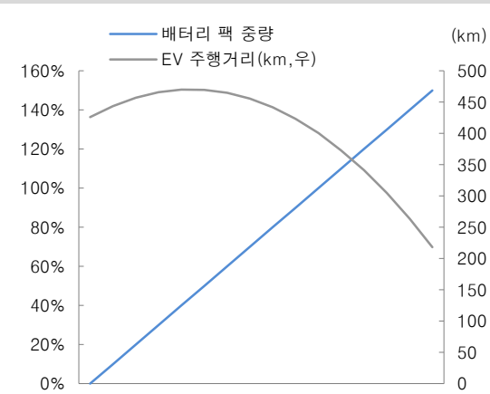
그림 35. 배터리 중량에 따른 EV 주행거리 향상 관계
