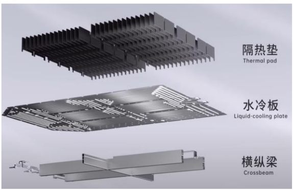
그림 4. CATL 기린 배터리
