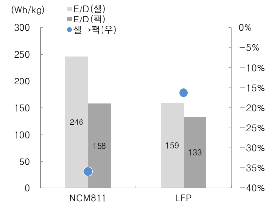
그림 11. 배터리 타입별 에너지밀도 차이 및 (셀→팩)손실
