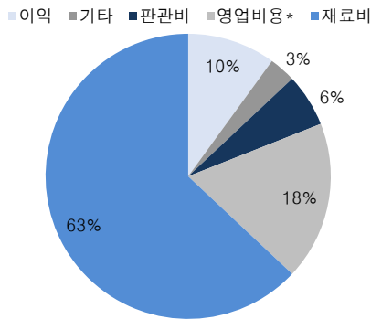
그림 29. EV 배터리 셀 원가구조
