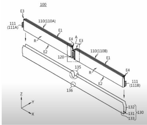
그림 15. LGES CTP 관련 특허: 파우치 셀
