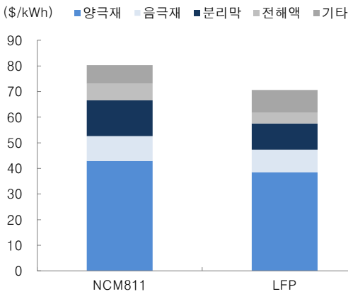
그림 30. LFP vs NCM 셀 재료비 원가구성
