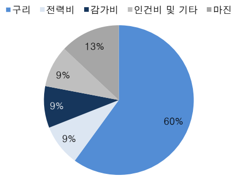
그림 164. 동박 원가구조
