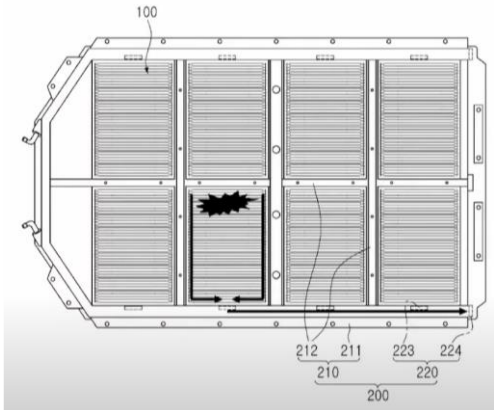
그림 21. SKOn CTP 관련 특허: 열/가스 분출
