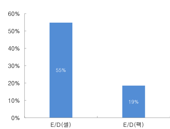
그림 12. LFP 대비 NCM811 에너지밀도 우위
