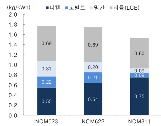
그림 69. 배터리 kWh 당 메탈별 소요량
