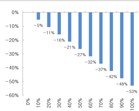
그림 36. 배터리 중량에 따른 EV 주행 효율 상관 관계
